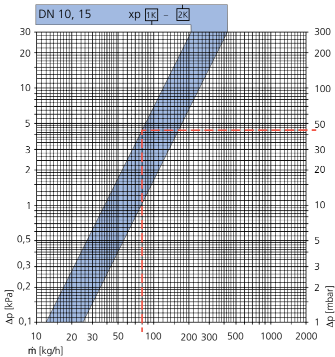
Diagramm DN 10 (3/8") und DN 15 (1/2"), Ventilunterteil mit Thermostat-Kopf
